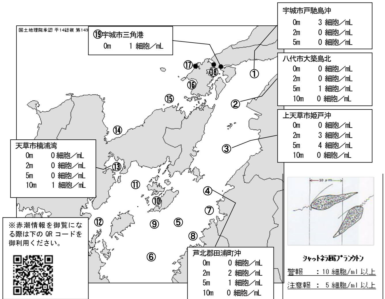
図 採水層別の海水1mlあたりのシャットネラ属の細胞数
